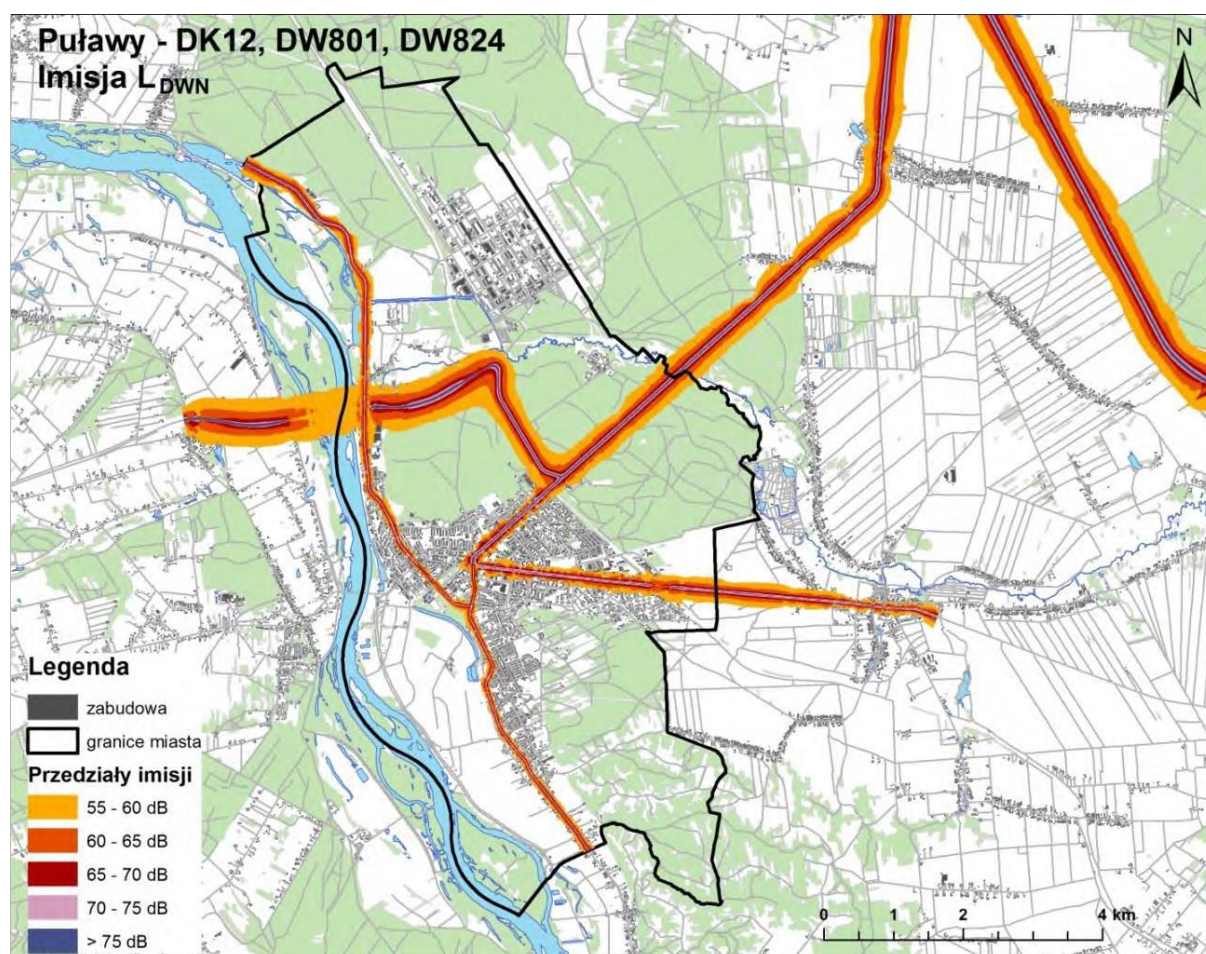
Ryc. 6. Mapa imisyjna LDWN odcinków DK 12, DW 801, DW 824 przebiegających przez Puławy (Raport oceny stanu klimatu akustycznego województwa lubelskiego na podstawie map akustycznych, WIOŚ, Lublin, 2018).
